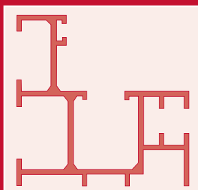
Coupe du rail haut et bas en Aluminium
