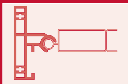
Vue en coupe des montants PVC
