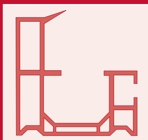
Coupe du rail haut et bas en PVC
