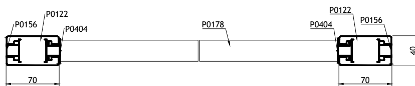
Section horizontale
