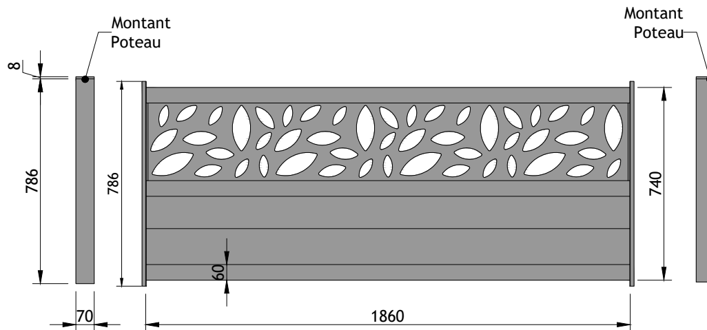
Vue en éclaté
